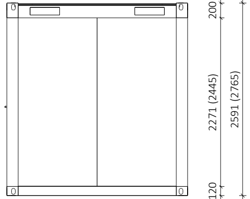
Ansicht von Rechts 1 : 50
